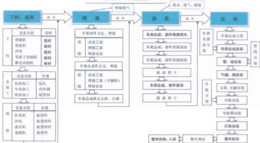
挂车生产工艺流程图
