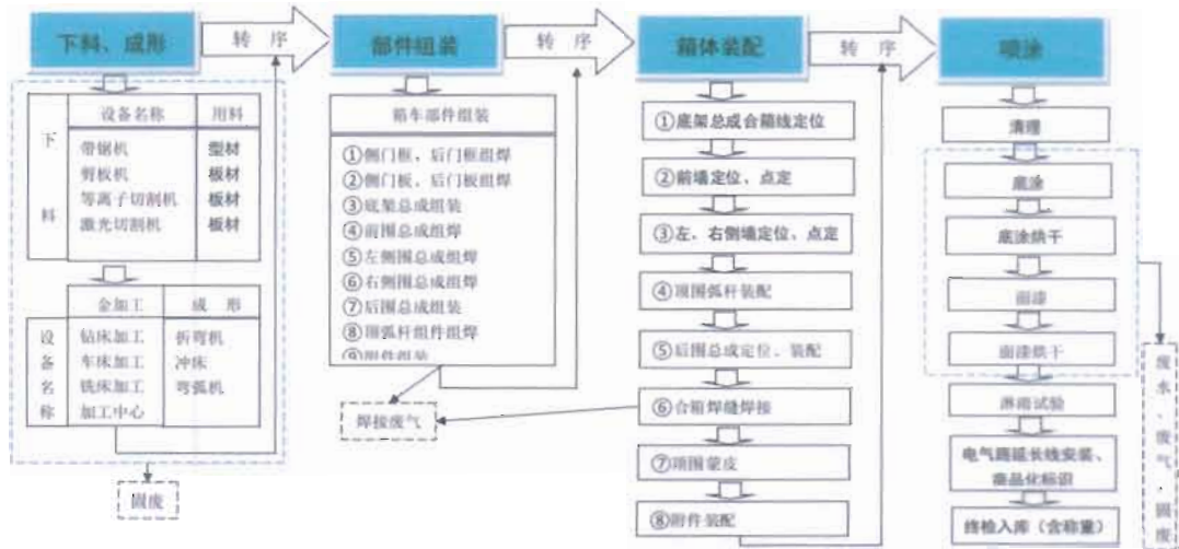
铝合金厢式车厢生产工艺流程图
