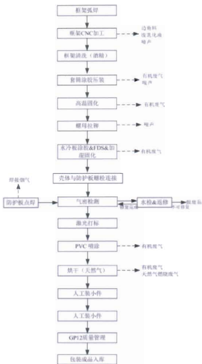
图 2-2 工艺流程图
